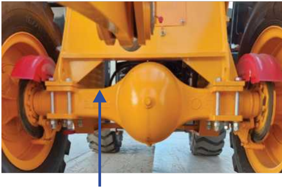
Respiradero de diferencial
